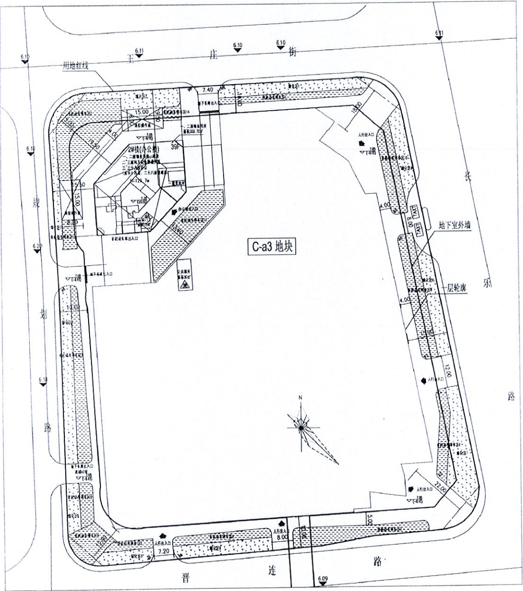
总平面图
